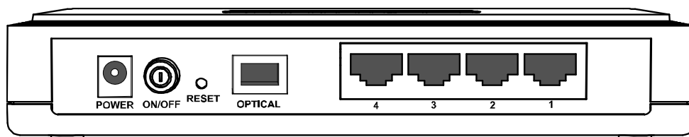
图 2-2 TL-EP140 后面板示意图
