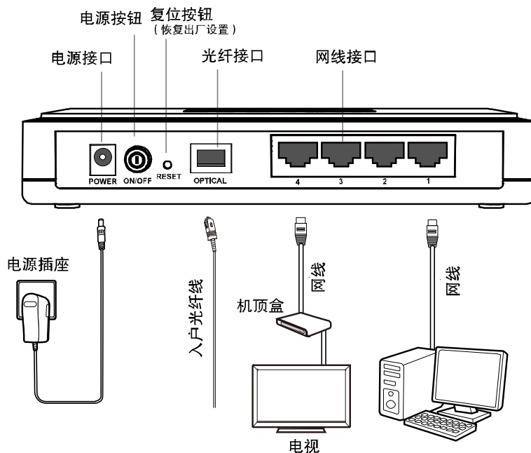
图 3-1 TL-EP140 硬件安装示意图
